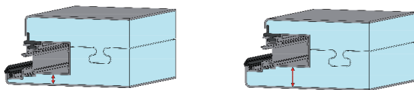
Coupe de SOLOBLOC 80.2, brevet \Omega méga et des différentes adaptations aux dormants
